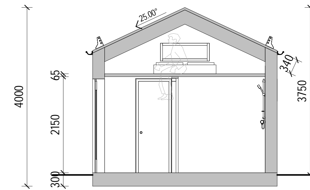
SEKTION A-A
