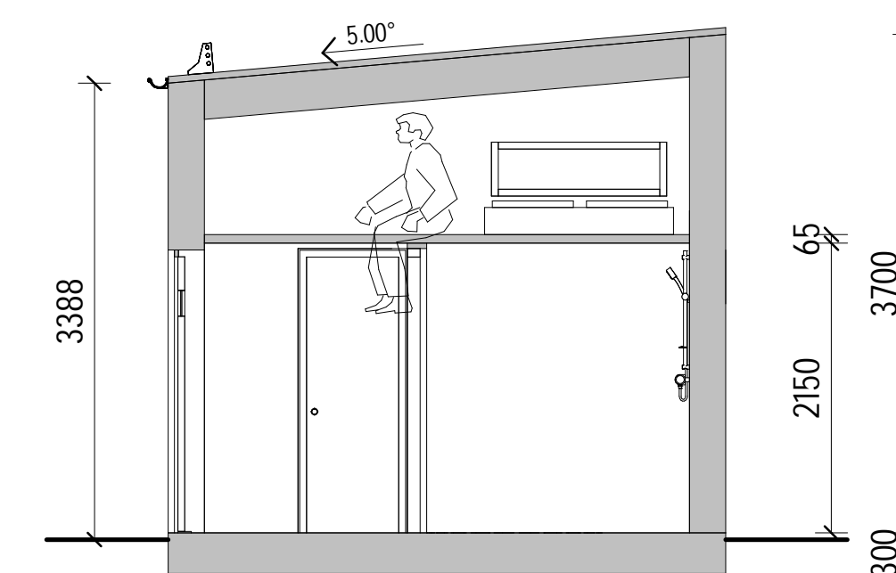
SEKTION A-A
