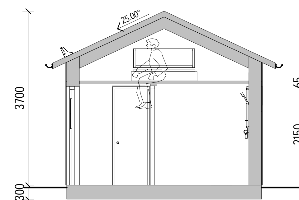
SEKTION A-A
