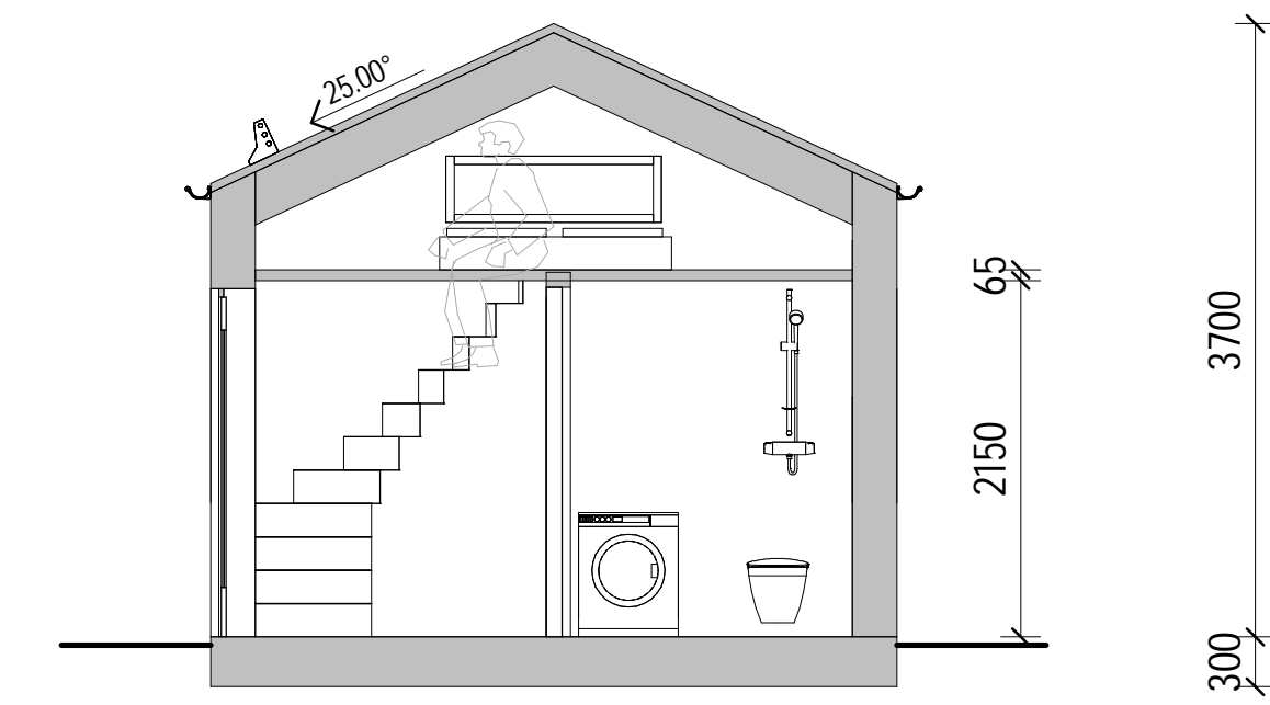
SEKTION A-A
