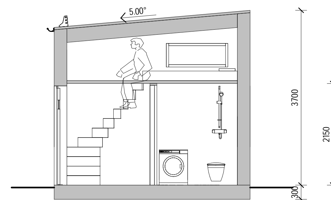
SEKTION A-A
