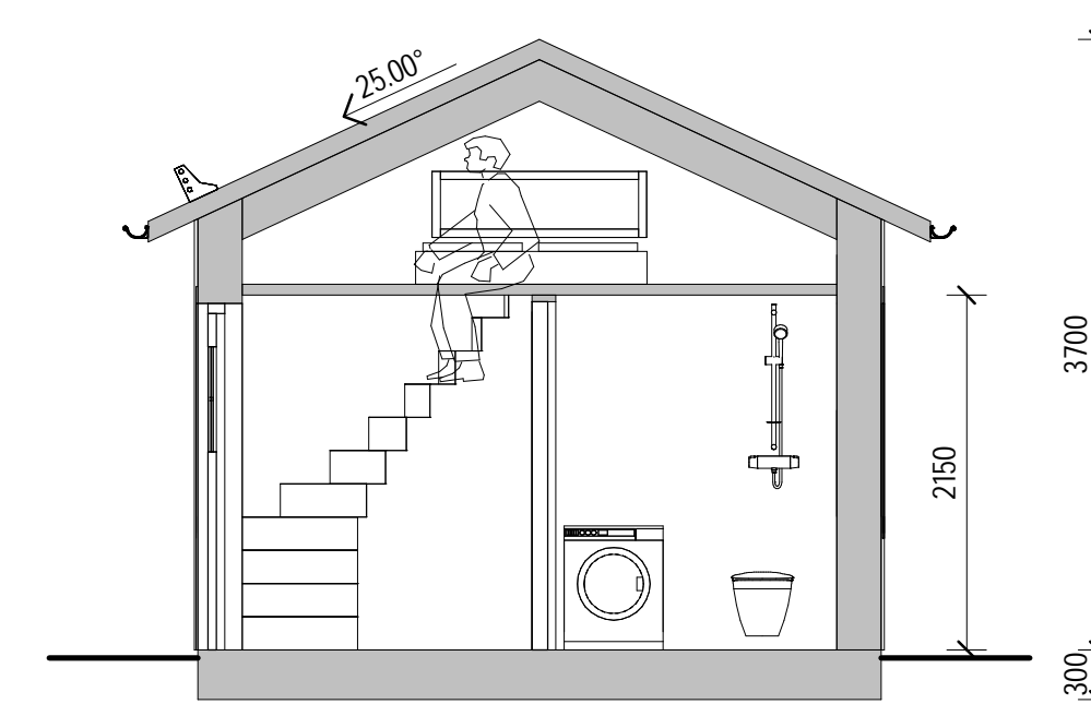
SEKTION A-A
