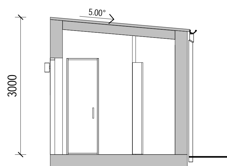
SEKTION A-A
