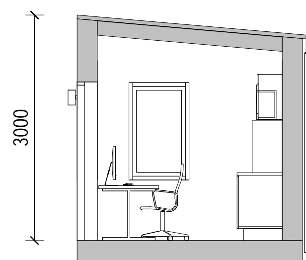
SEKTION A-A
