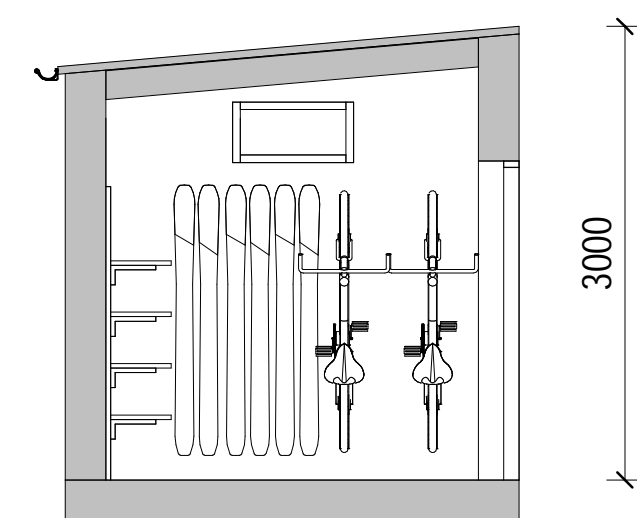
SEKTION A-A
