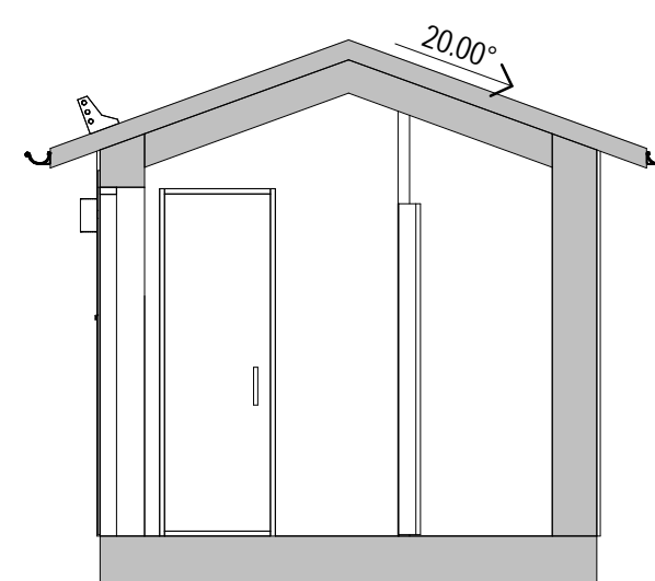
SEKTION A-A
