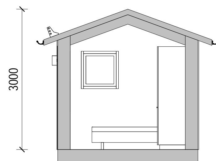
SEKTION A-A
