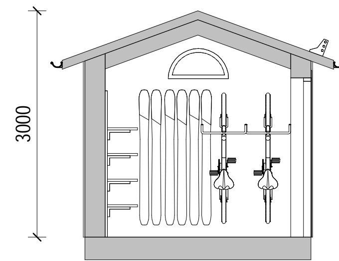
SEKTION A-A
