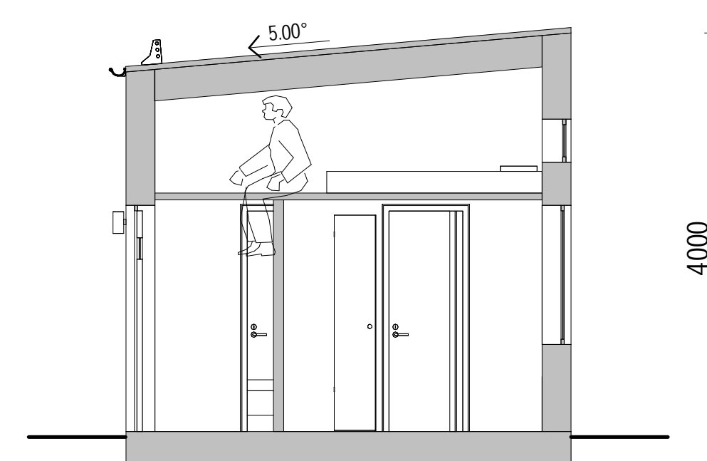
SEKTION A-A
