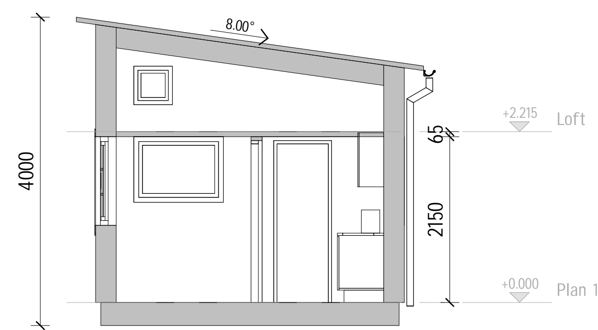
A-A
