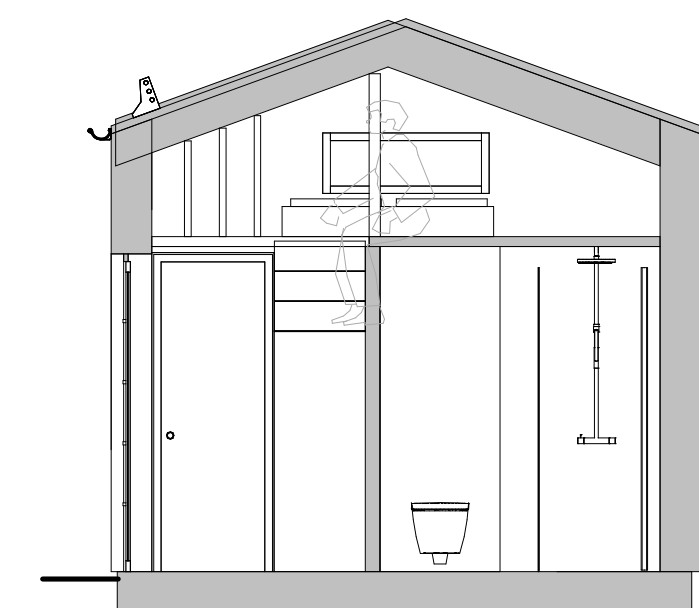
SEKTION A-A
