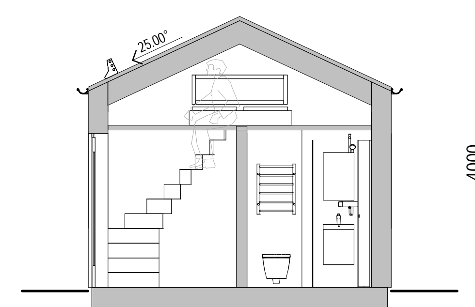
SEKTION A-A
