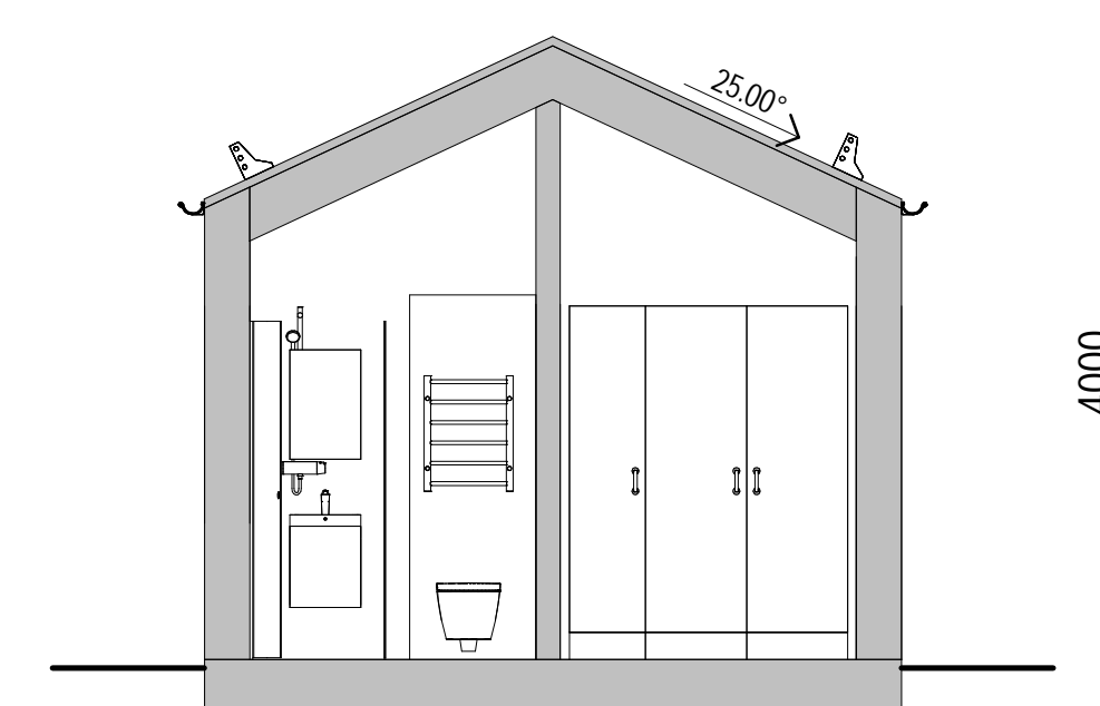
SEKTION A-A
