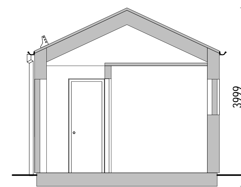
SEKTION A-A
