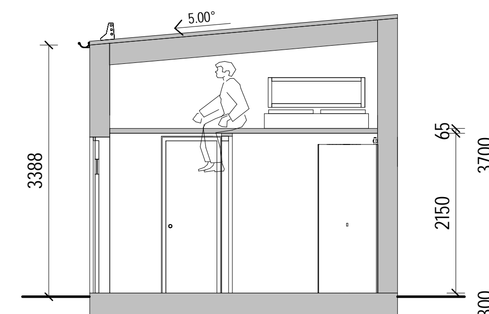
SEKTION A-A
