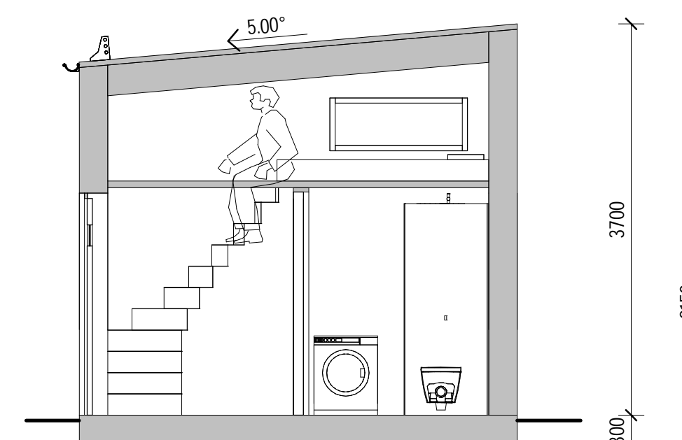
SEKTION A-A
