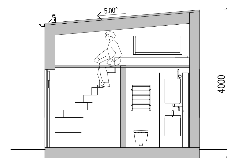
SEKTION A-A
