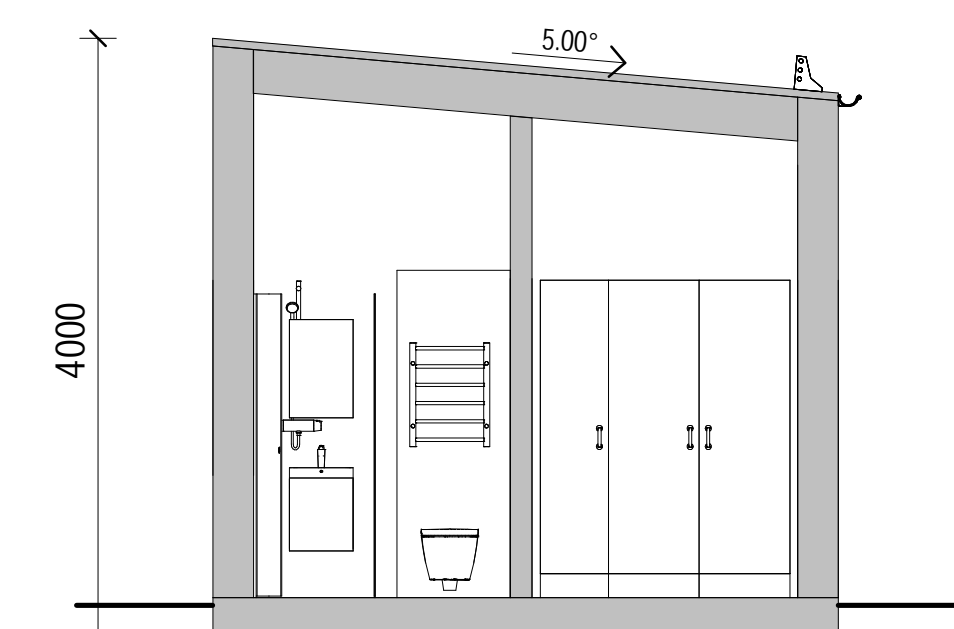
SEKTION A-A
