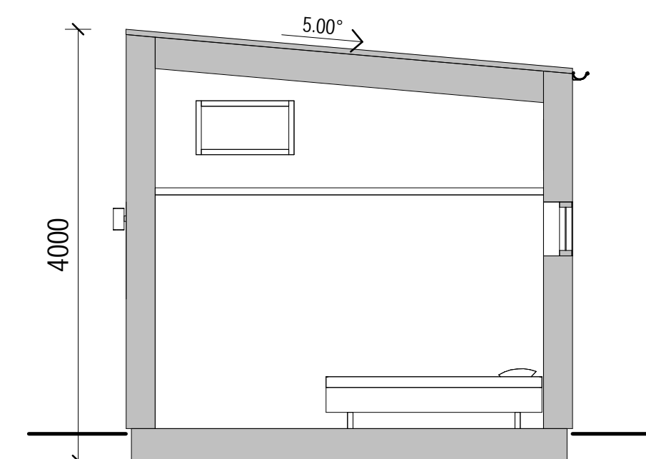
SEKTION A-A
