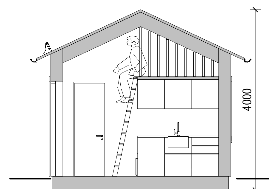
SEKTION A-A
