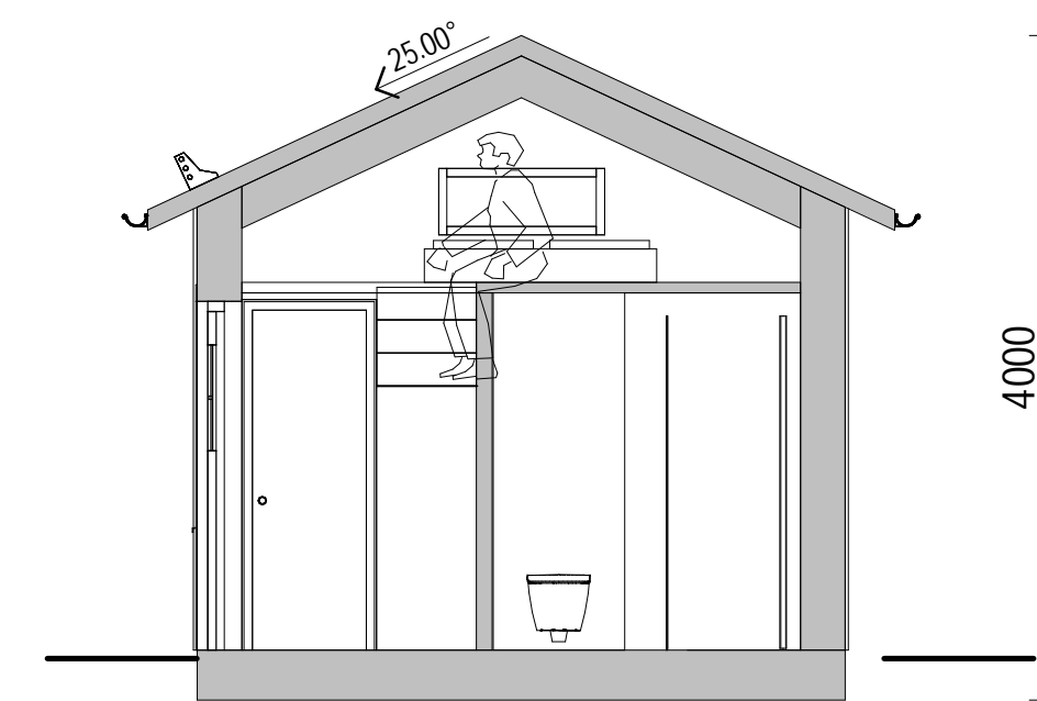
SEKTION A-A
