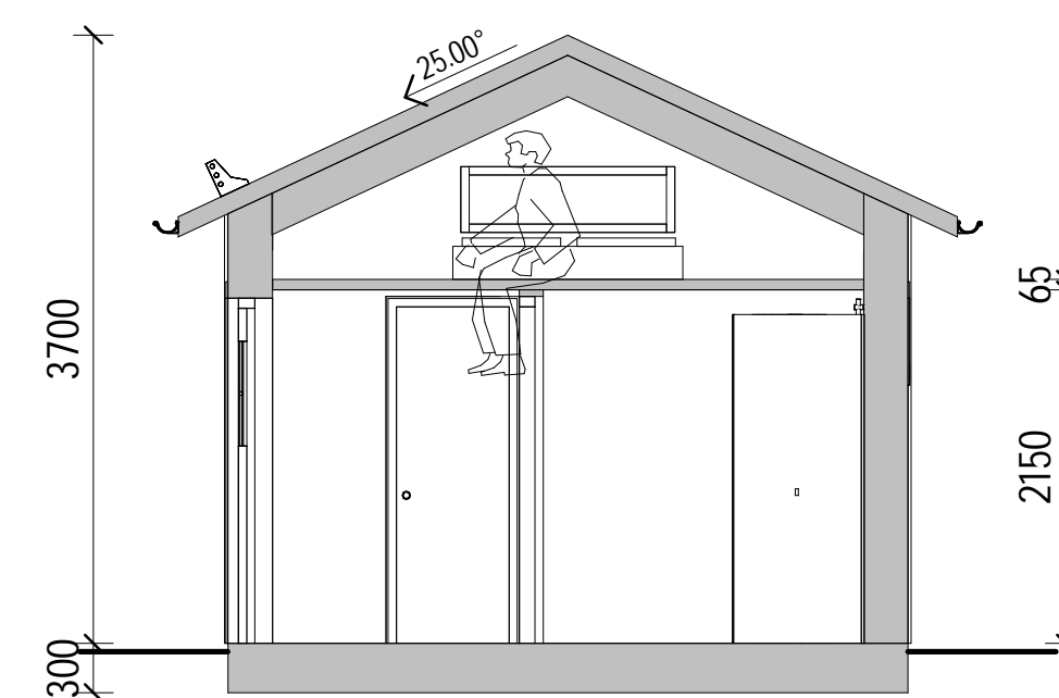
SEKTION A-A
