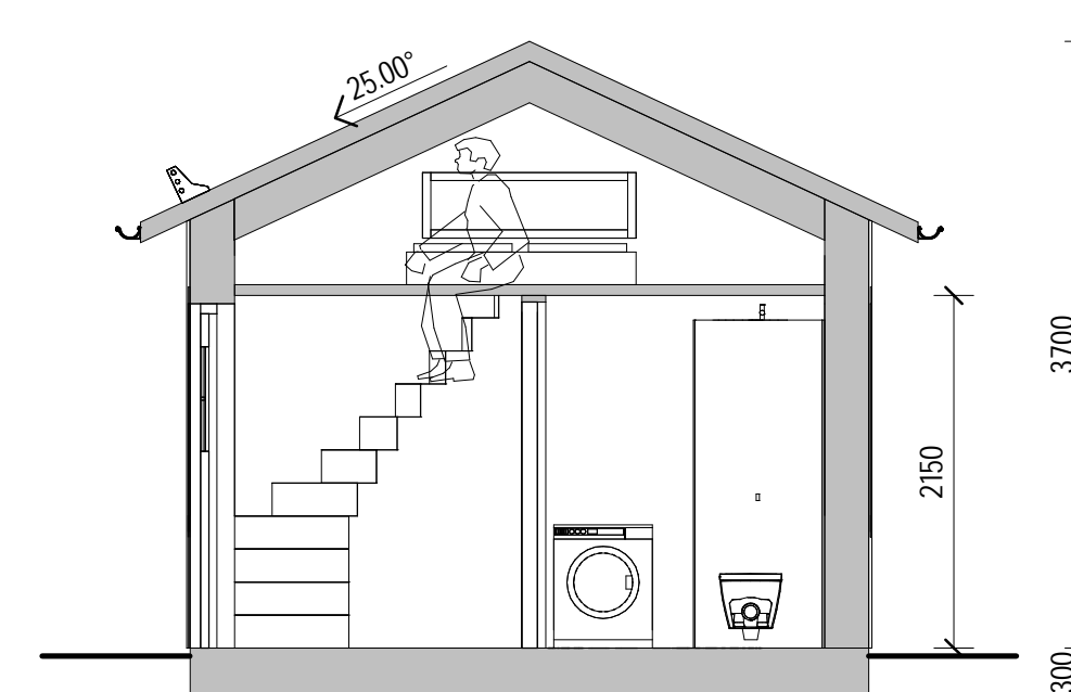
SEKTION A-A
