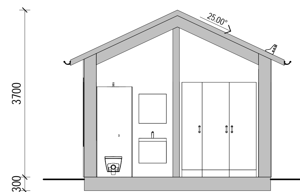
SEKTION A-A
