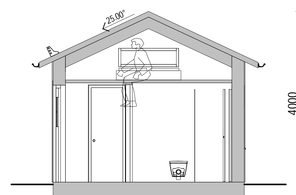
SEKTION A-A
