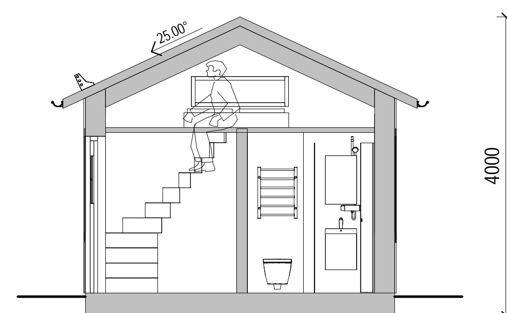
SEKTION A-A
