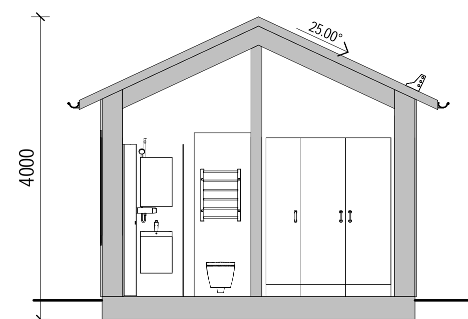
SEKTION A-A
