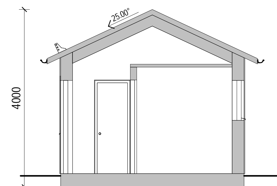
SEKTION A-A
