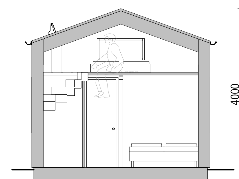
SEKTION A-A
