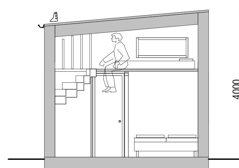
SEKTION A-A
