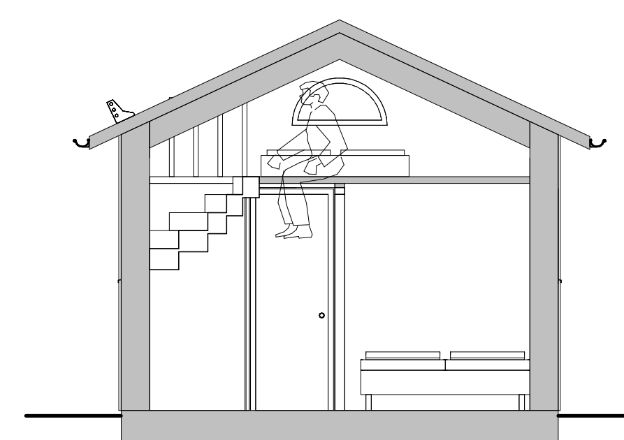
SEKTION A-A
