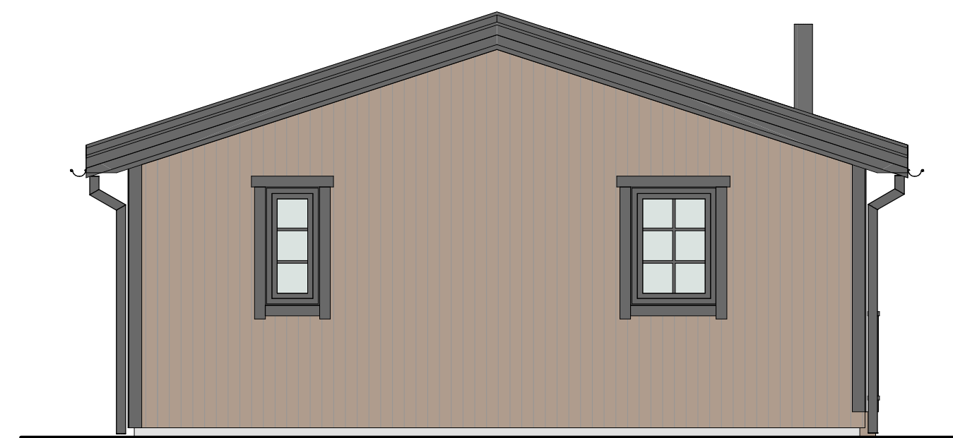
FASAD SIDA 1
