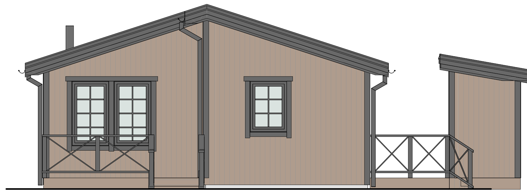
FASAD SIDA 1
