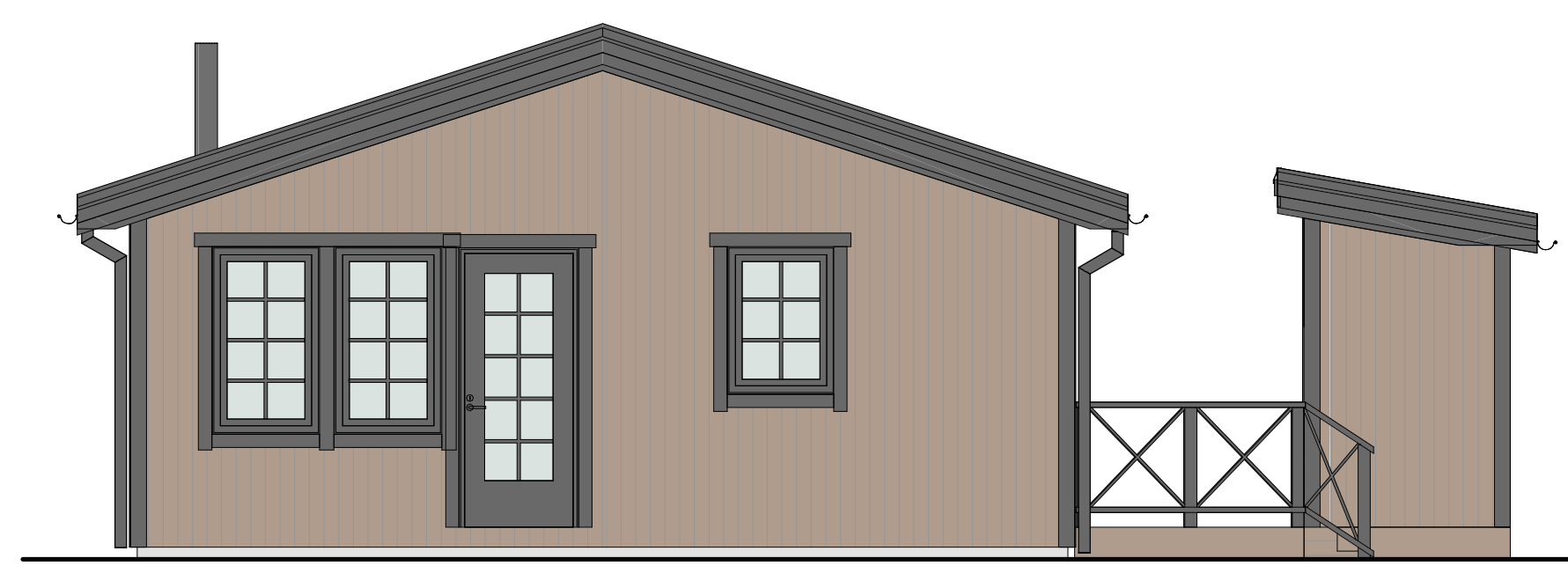
FASAD SIDA 1
