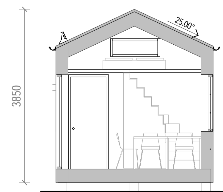
SEKTION A-A
