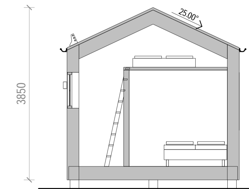
SEKTION A-A
