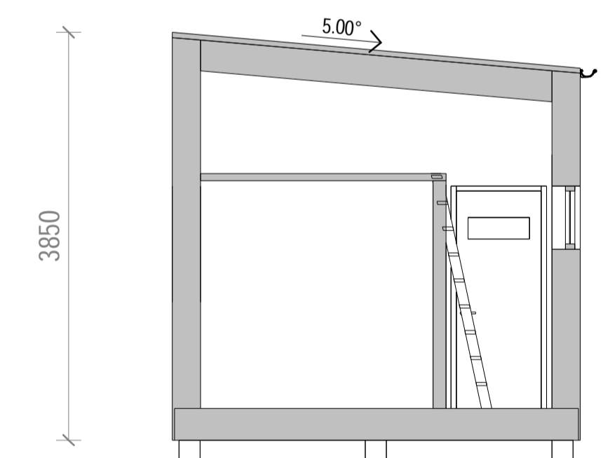
SEKTION A-A
