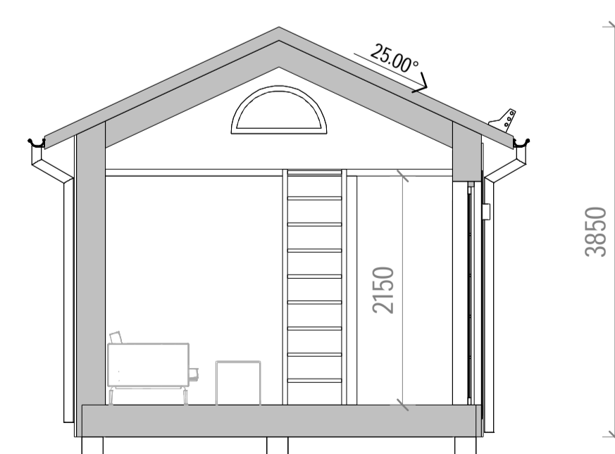
SEKTION A-A
