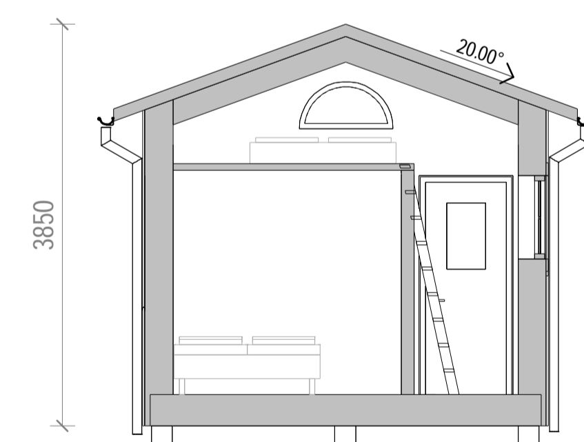
SEKTION A-A
