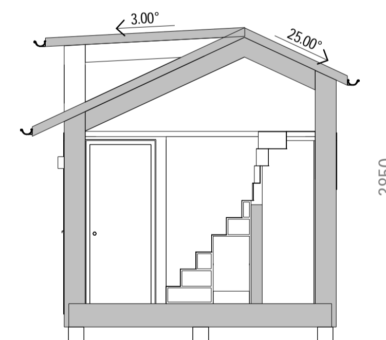
SEKTION A-A
