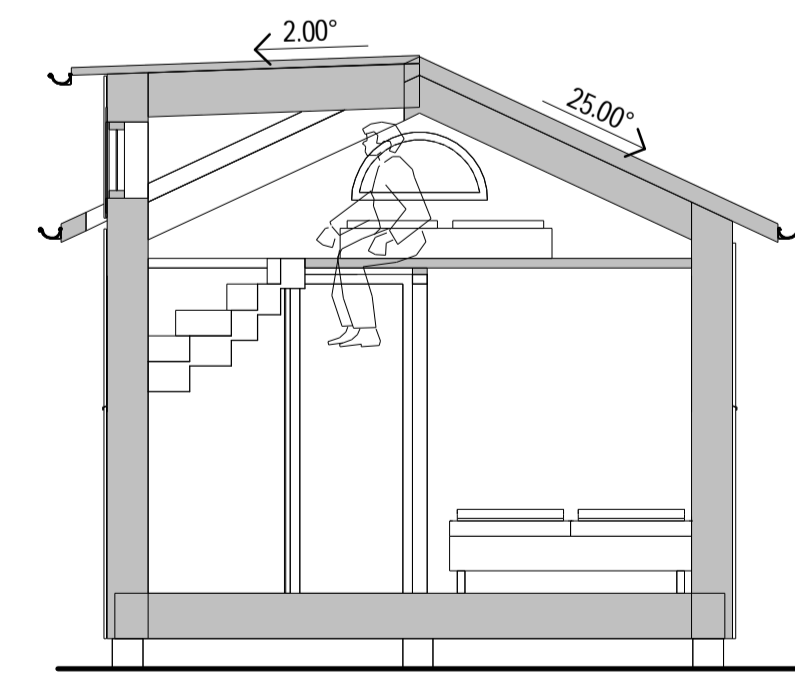
SEKTION A-A
