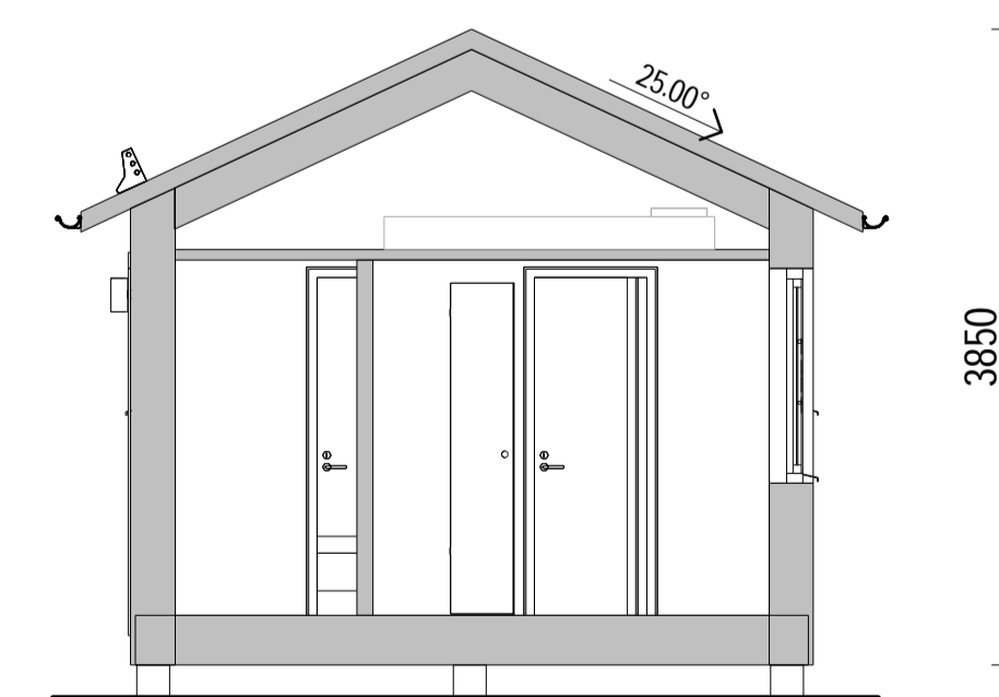
SEKTION A-A
