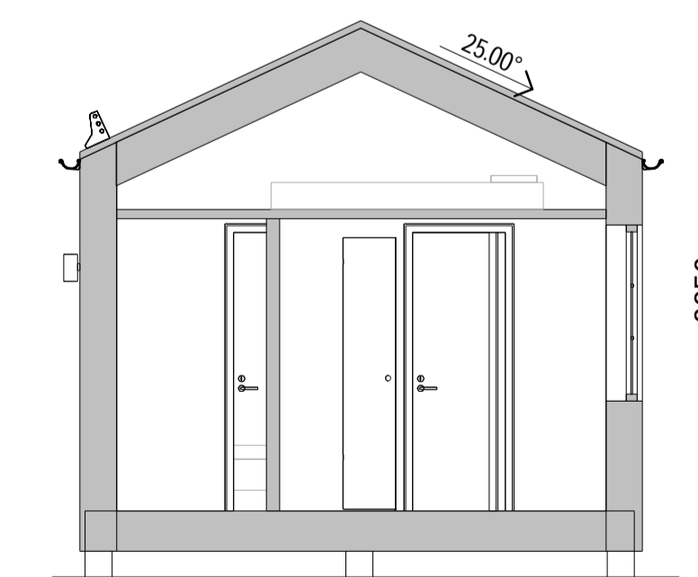
SEKTION A-A
