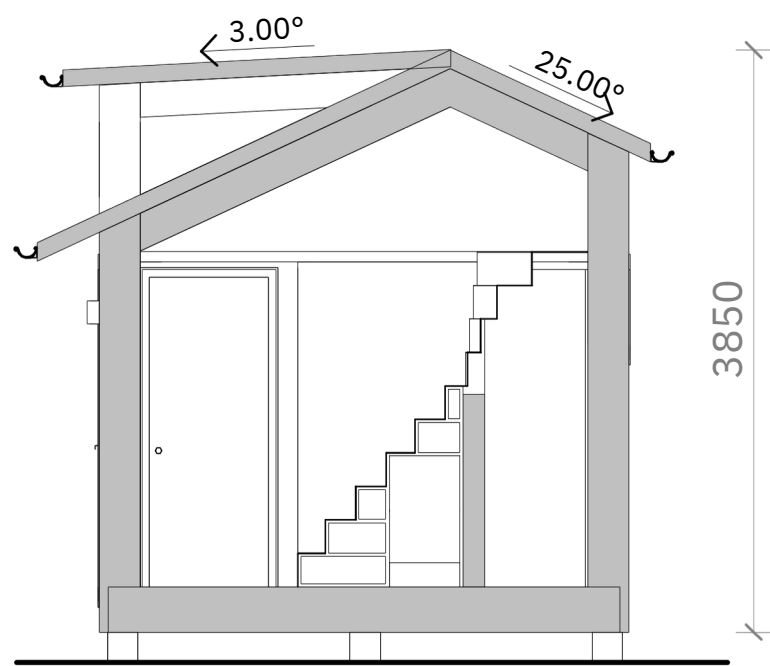
SEKTION A-A
