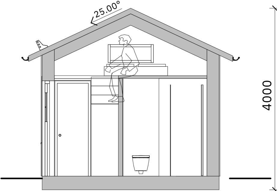
SEKTION A-A
